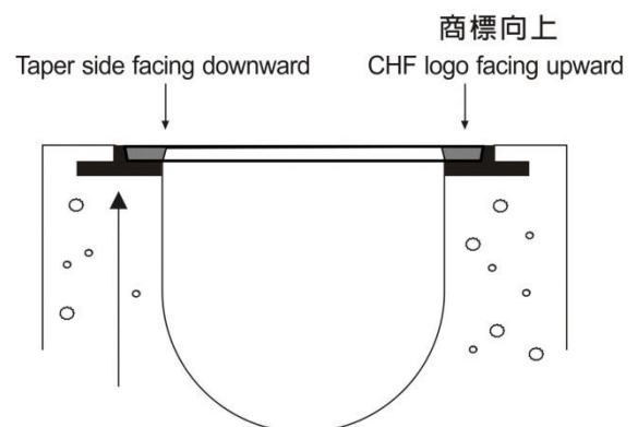
生鐵 T 型角鐵裝置圖
